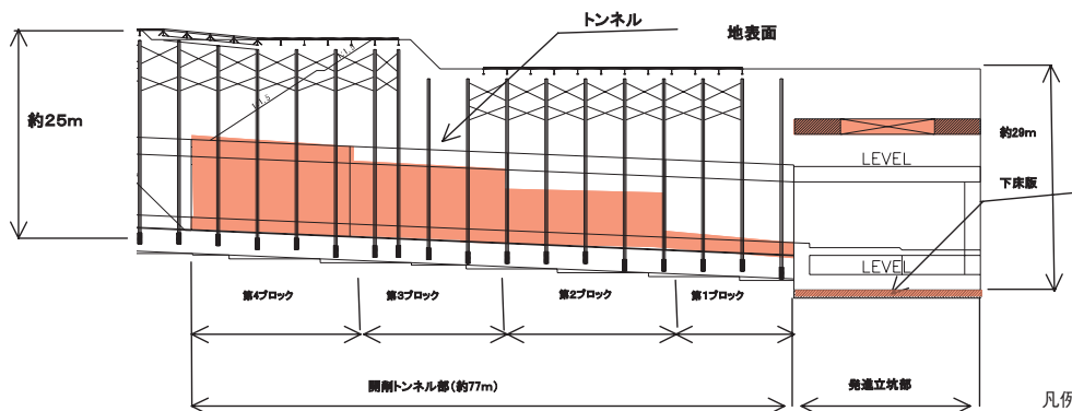
開削トンネル部 (A-A断面)
