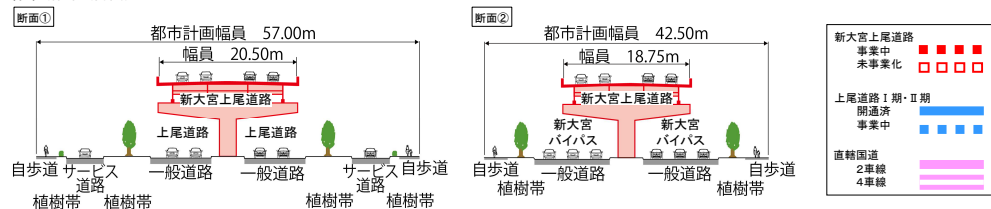
標準断面図（計画）
