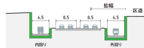
擁壁・掘削 C-C横断模式図
