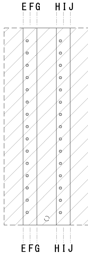
【D - E - F - G - H - I - J - K線組合せ参考断面図】
